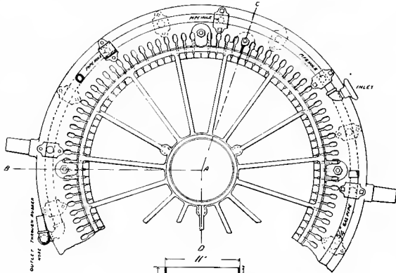
Fig. 5365. Plan.
